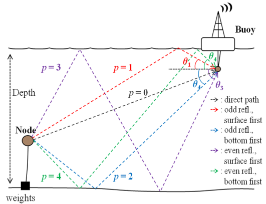
그림 2. 수중채널에서의 다중경로
