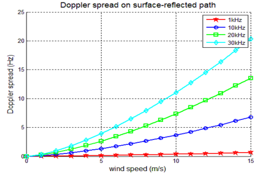
그림 1. 해면 반사에 의한 도플러 확산
