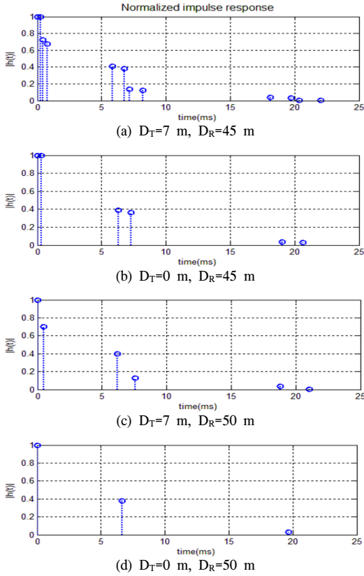
그림 5. 모의 수중채널의 임펄스 응답
