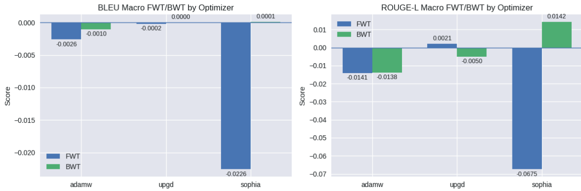
그림 1 급격한 도메인 및 언어 변화 환경에서 옵티마이저에 따른 Blue 와 Rouge-L 에 따른 BWT, FWT 의 평균값
